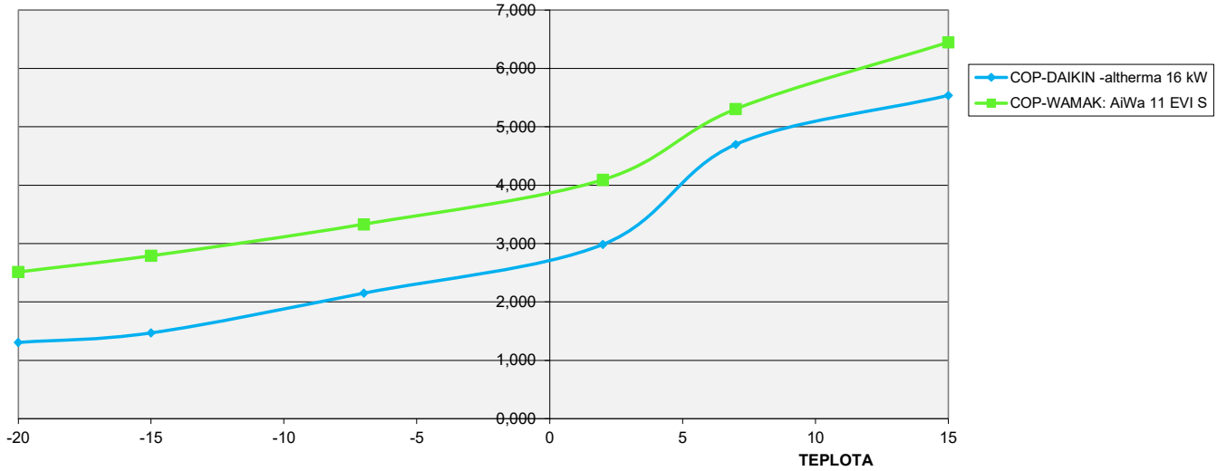
COP pri teplote vykurovacej vody 35°C (kW)
